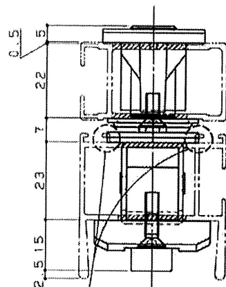
店舗引戸 (1980~1987)
